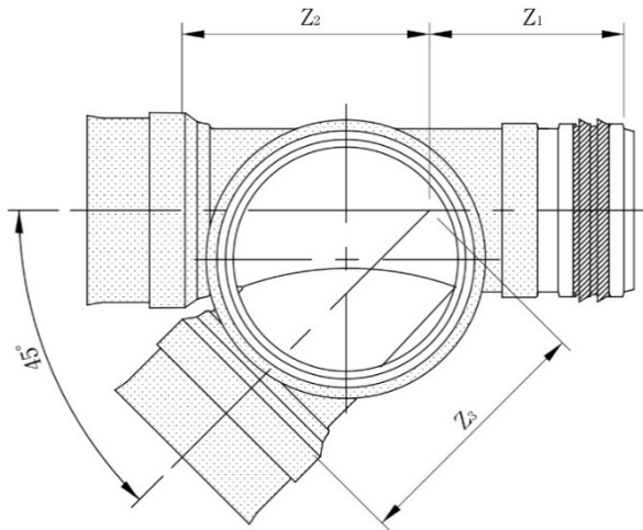
標準受口形
