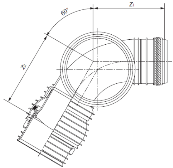
自在受口形
