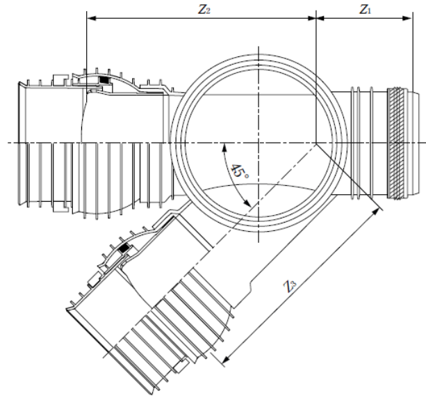
自在受口形
