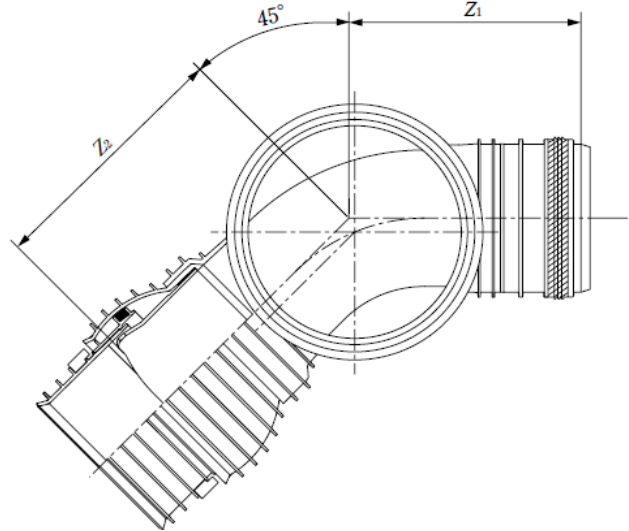
自在受口形
