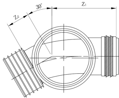
標準受口形
