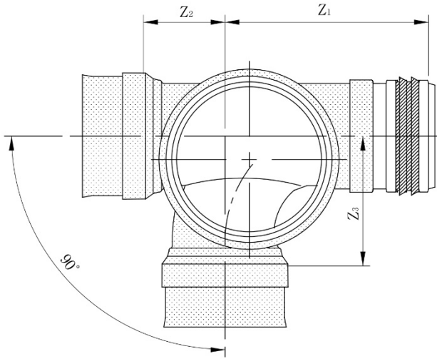
標準受口形
