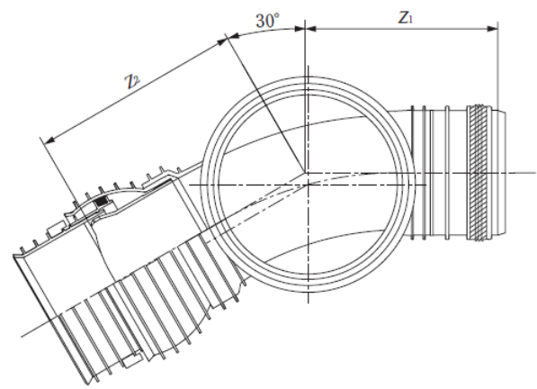
自在受口形
