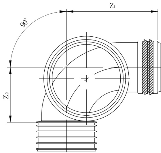
標準受口形
