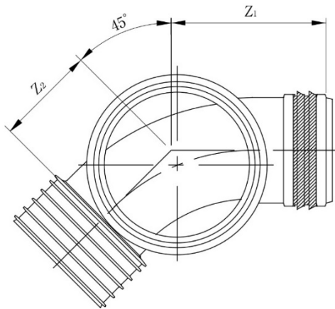
標準受口形
