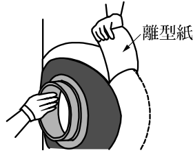
図7-69 コンクリート製マンホールへの接合
