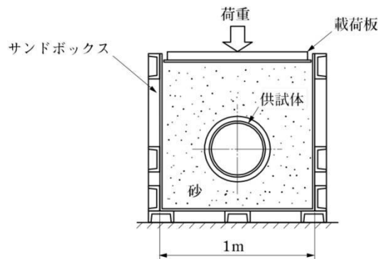
図8-1 サンドボックス実験装置
