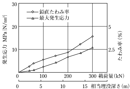
図8-5 載荷荷重と発生応力、たわみの関係 (砂質土)
