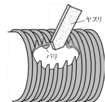
図7-13 ばり取り
