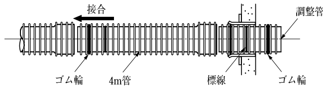
図7-37 本管の接合
