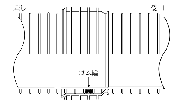
図7-9 ゴム輪接合例
