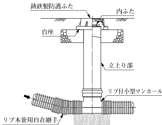
図 5-2 リブ本管自在継手を用いる場合
