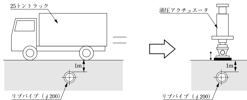
図8-12 実験モデル
