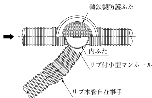
図3-23 管路の合流
