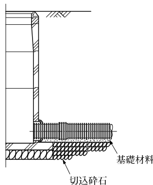
図7-53 コンクリート製マンホール余掘り部の埋戻し
