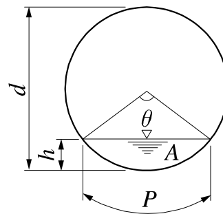
図 3-1 流水断面
